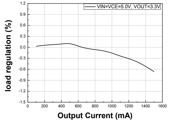
16、负载调整率 @ VOUT=3.3V
