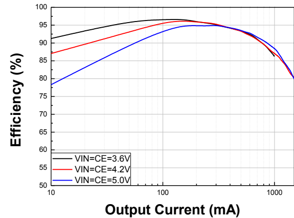
12、效率 @ VOUT=3.3V
