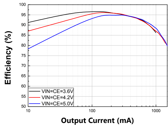
12、效率 @ VOUT=3.3V
