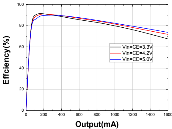
5、效率 @ VOUT=1.2V
